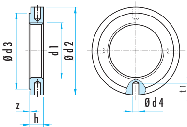
DIN 1816
