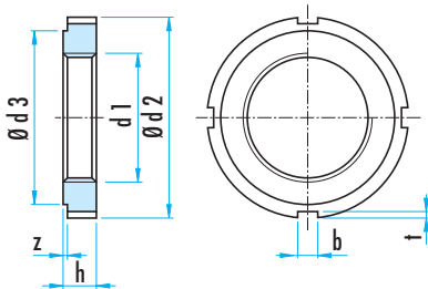
DIN 1804
