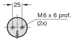
Vue selon X
