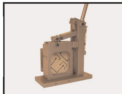
Art. TAT.30005 Cisaille pour 4 dimensions de profilés pour canaux de câbles avec système de butée avec latte graduée. Poids : 22 Kg
