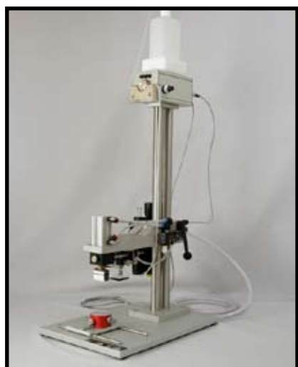
Unité pneumatique avec pompe
