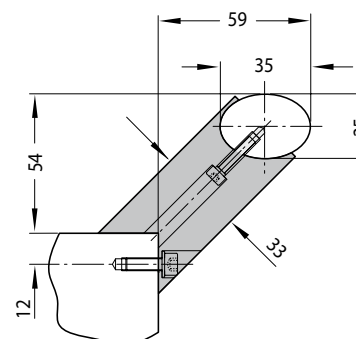
RSC.U4.35 horizontale montage
